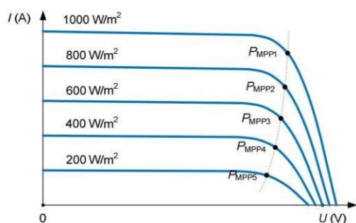
Slika 3.9. Utjecaj povećanja intenziteta zračenja na I-U karakteristiku [8]
