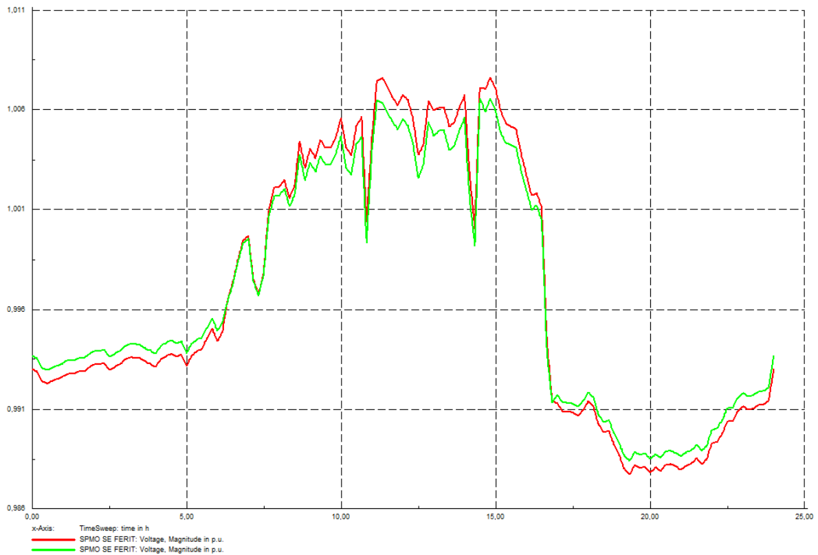
Slika 5.26. Promjena napona na 0.4 kV sabirnici (c-bez baterije, z-s baterijom)
