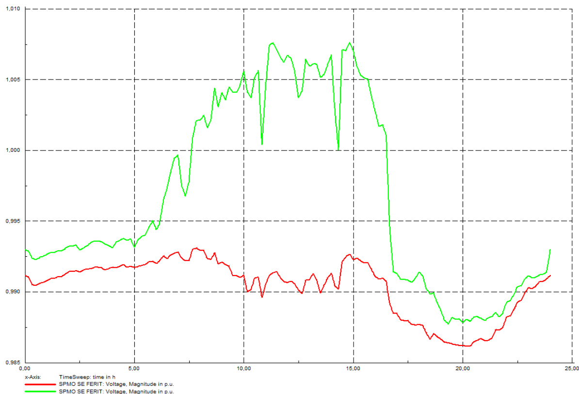
Slika 5.4. Promjena napona na sabirnici SPMO (c-prije integracije, z-nakon integracije)
