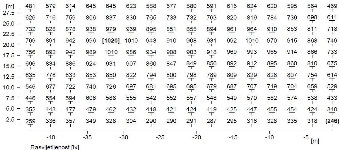
Slika 6.6. Brojčani prikaz rasvijetljenosti cijeloga terena uz tribine
