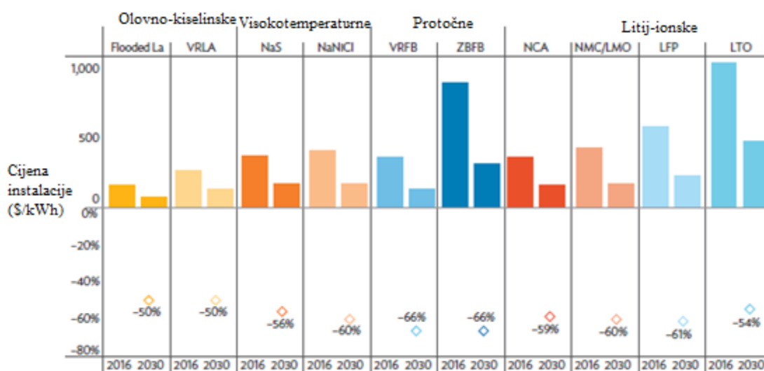
Slika 4.7. Usporedba cijene baterijskih spremnika 2016. i očekivane cijene 2030. godine
