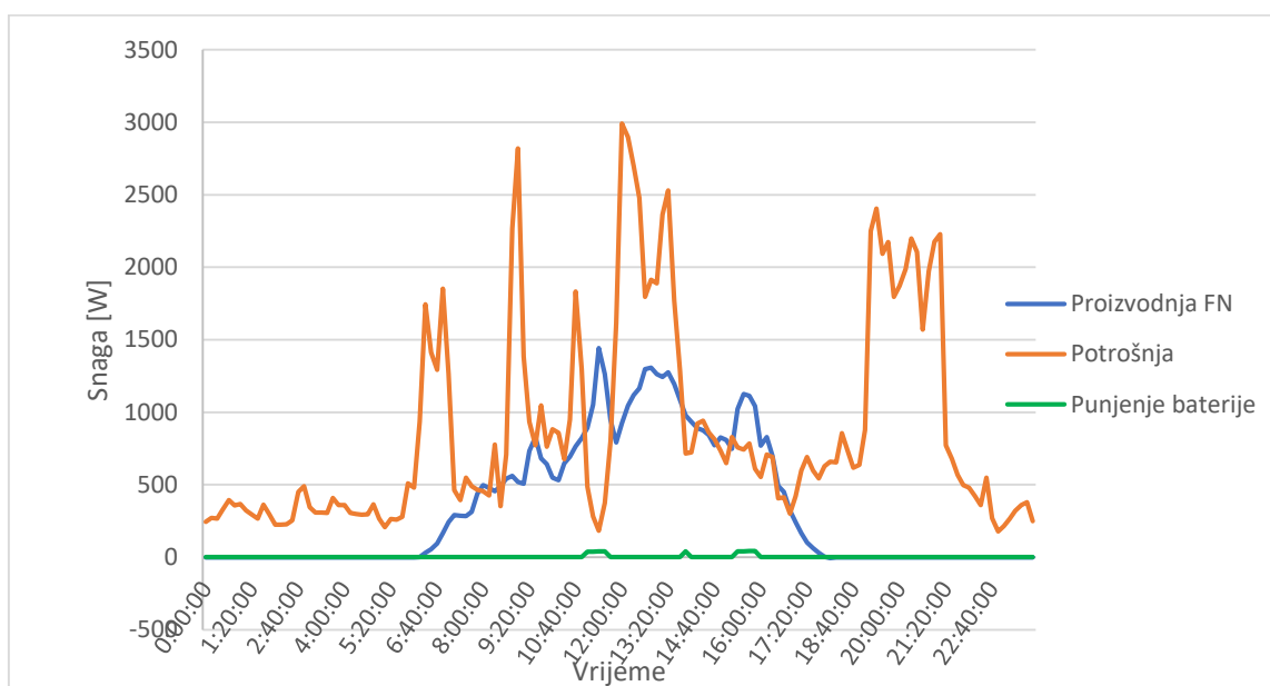
Slika 5.10. Graf proizvodnje FN-a, potrošnje kuće i punjenja baterije
