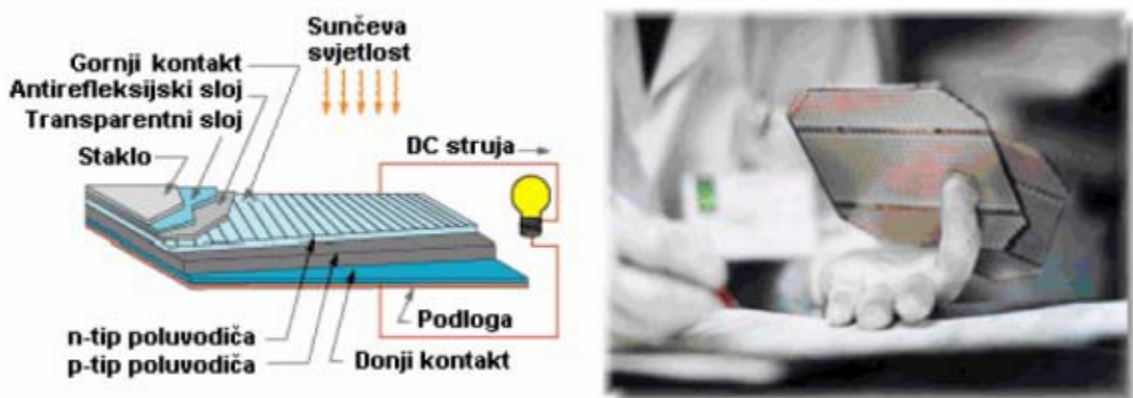
Slika 2.7. Monokristalne ćelije, [2].
