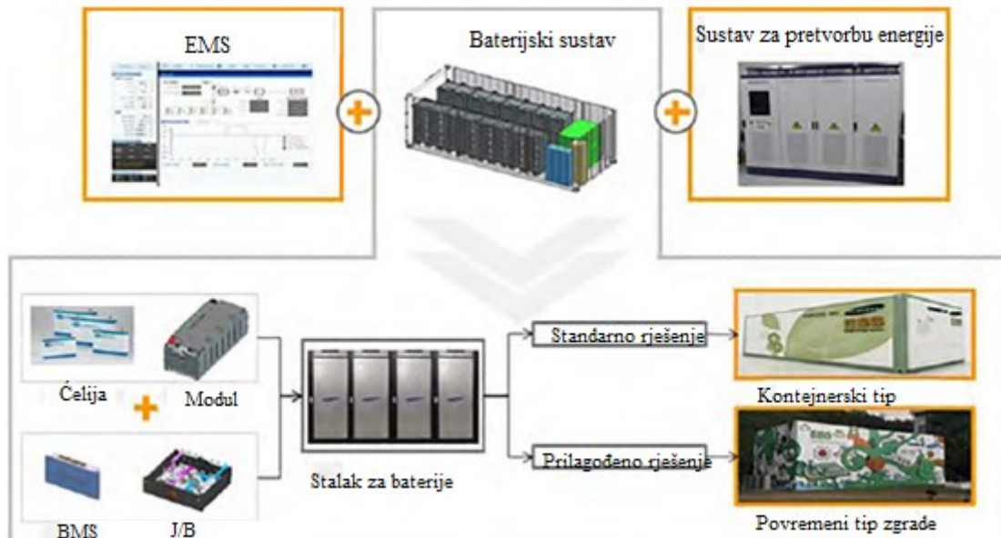
Slika 4.6. Shematski prikaz baterijskog sustava za pohranu energije, [11].
