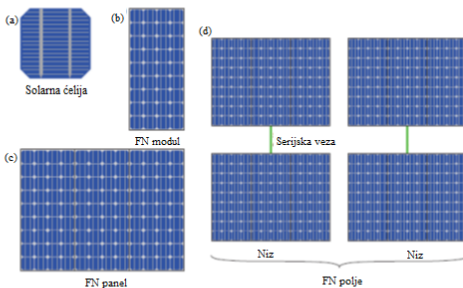
Slika 2.9. Ilustracijski prikaz (a) solarne ćelije, (b) FN modula, (c) FN panela i (d) FN polja
