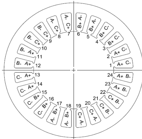
Slika 3.2.1 Trofazni stator sinkronog reluktantnog motora [10]
