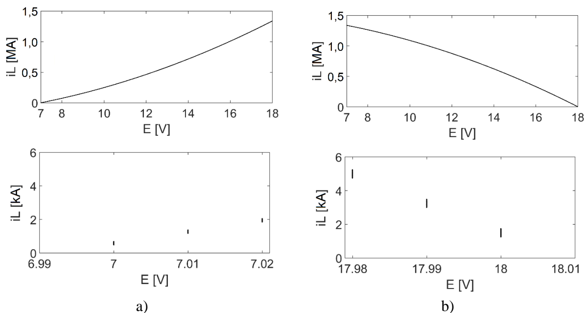
Slika P 2.3 Bifurkacijski dijagrami i_L = f(E) uzlaznog pretvarača za U_{dt} = -1 V uz a) povećavanje ulaznog napona, b) smanjivanje ulaznog napona.
