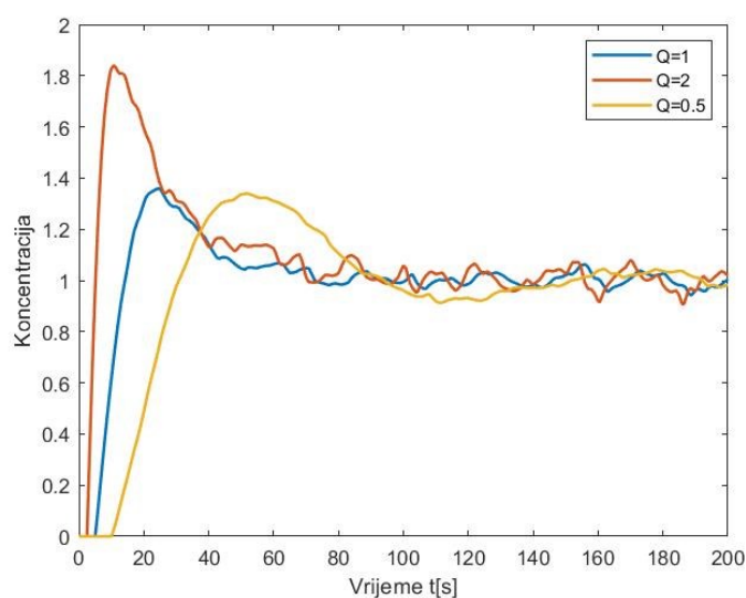
Sl. 4.9. Prikaz odziv jedнопетлјасте структуре управљања pod utjecajem smetnje.
