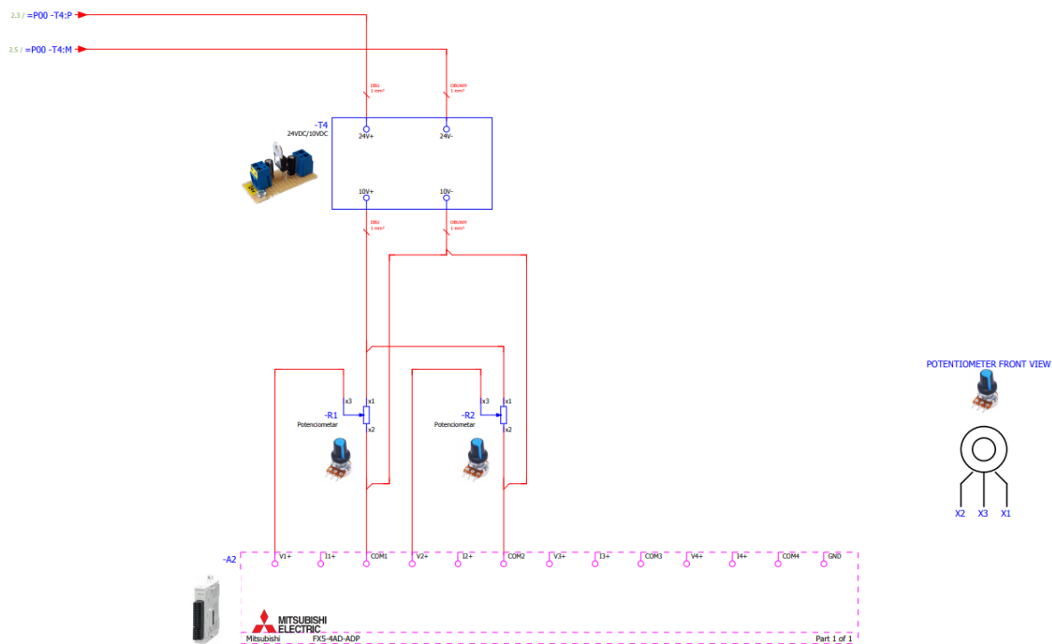
Sl. 2.12 Električna shema spajanja potenciometra na FX5-4AD-ADP [4]
