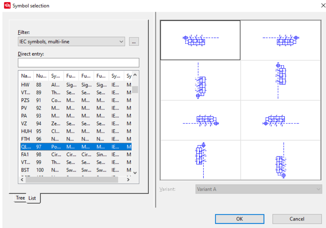
Slika 3.178. Izbornik simbola
