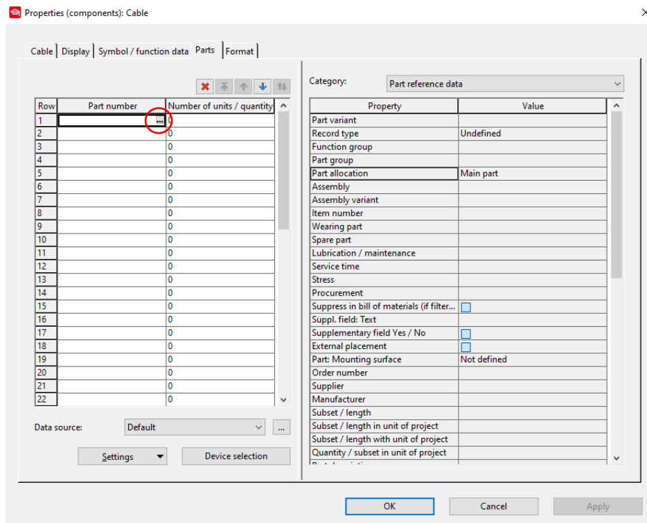
Slika 3.250. Kartica "PARTS"
