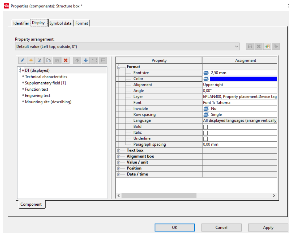
Slika 3.141. Kartica "DISPLAY"
