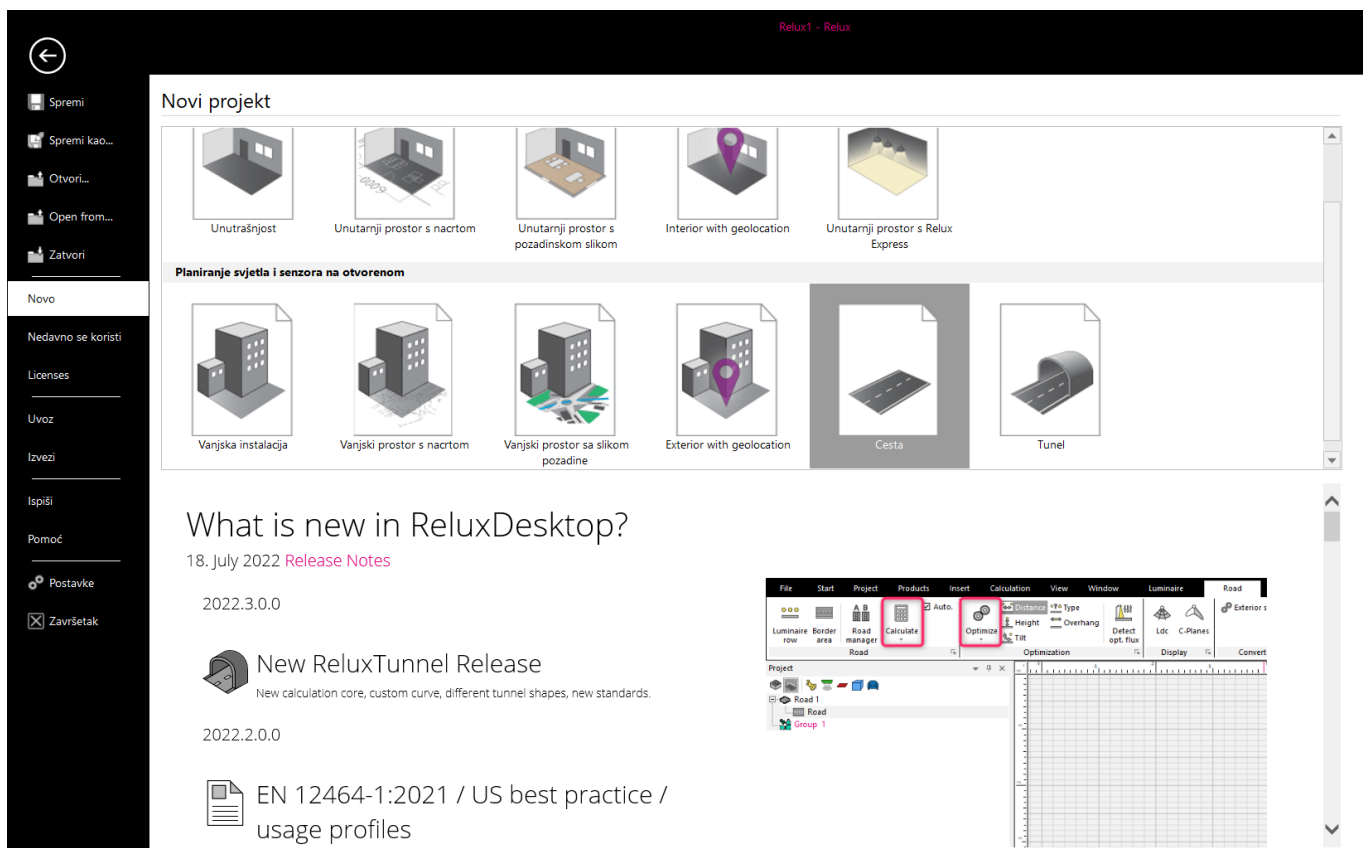
Slika 4.1. Program Relux
