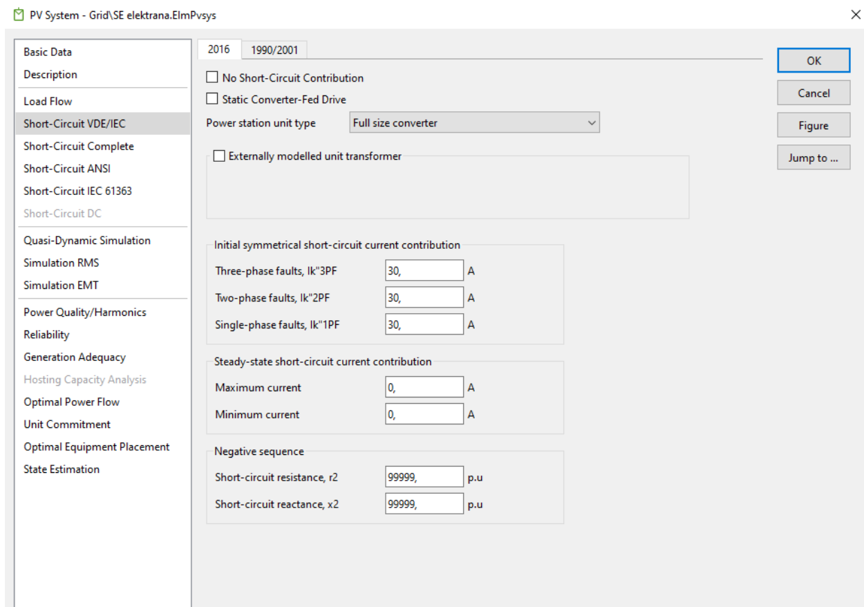
Slika 4.10. Prikaz kartice Short-Circuit VDE/IEC [11]
