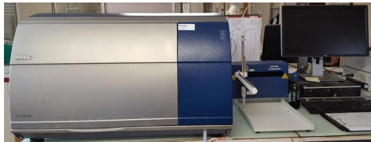
Sl. 2.1. Laboratorijski instrument za mjerenje parametara vina tvrtke Foss, model WineScan TM SO 2 .
