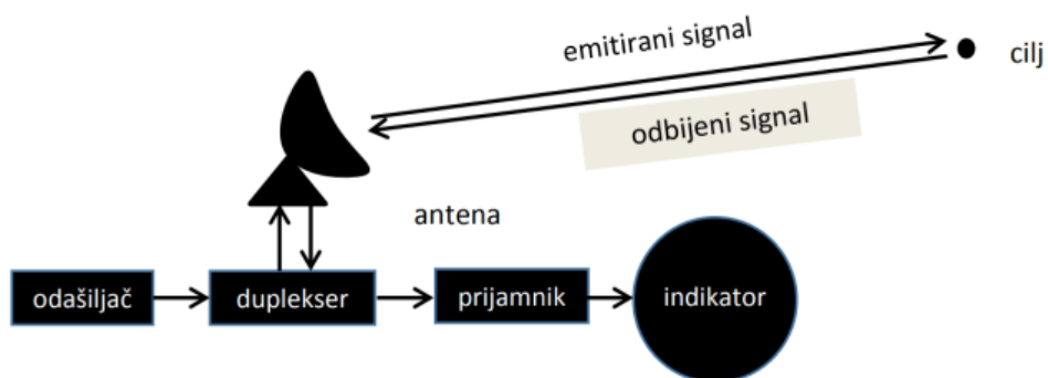
Slika 2.3. Blok dijagram Radara[13]
