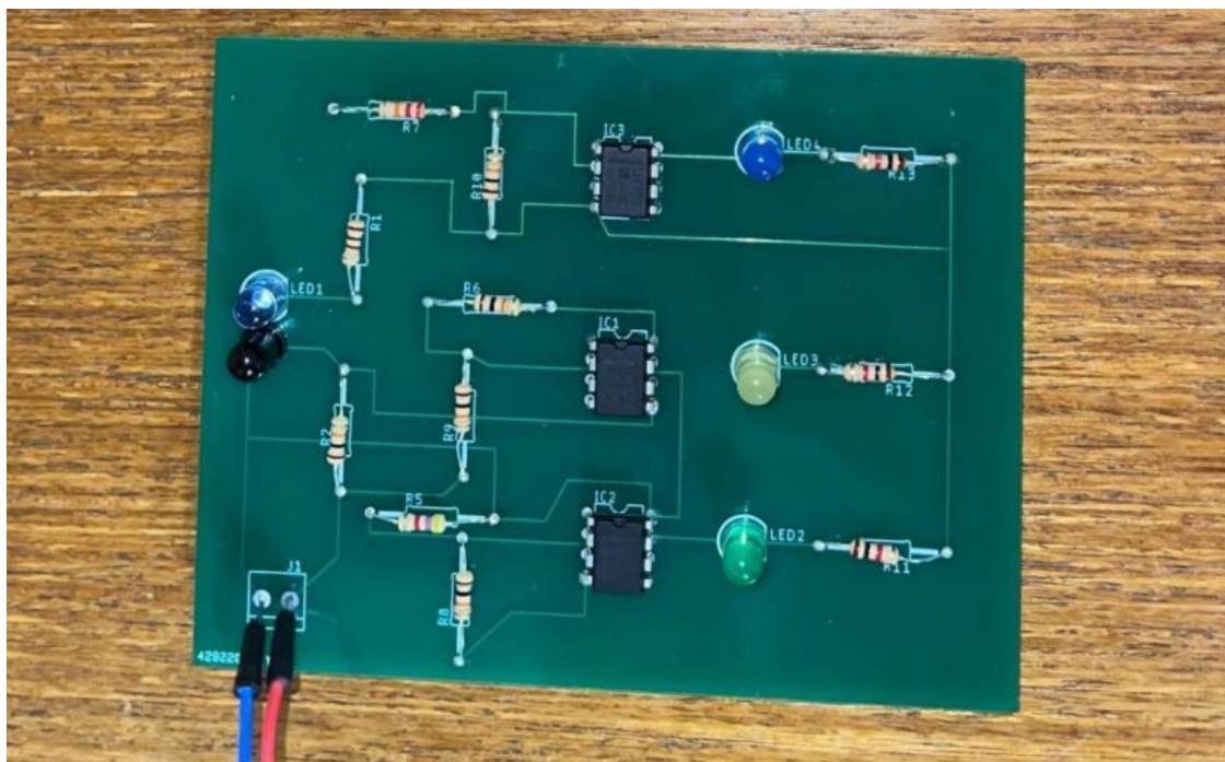
Slika 3.5. Prikaz uređaja za mjerenje udaljenosti zasnovanog na IR senzoru izrađenog na PCB pločici
