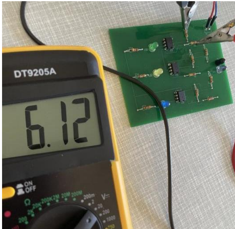
Slika 4.3. Rezultat mjerenja referentnog napona na otpornicima R5 i R9
