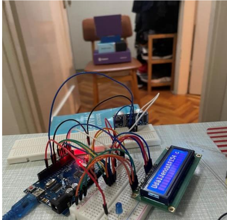
Slika 4.30. Mjerenje udaljenosti od objekta kartonske površine veličine 17x23 cm
