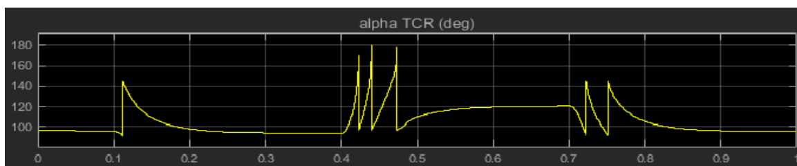
Slika 5.3.: Valni oblik faktora snage na TCR grani
