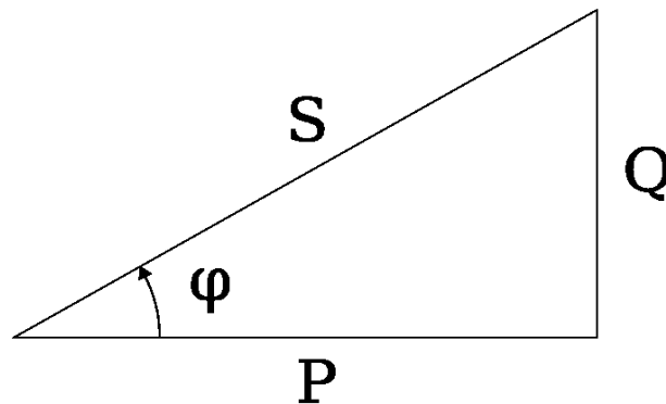
Slika 2.3.: Trokut snage [4]
