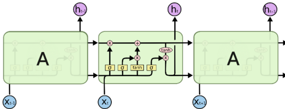
Slika 4.21. LSTM modul.
