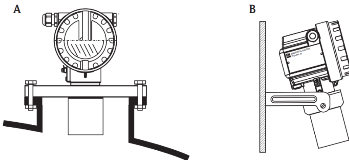
Slika 7.2. Načini postavljanja mjernog uređaja Prosonic FMU44
