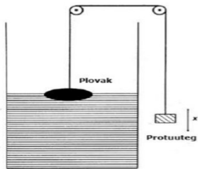
Slika 2.2. Prikaz mjernika s plovkom i formulu za izračun parametara plovka [6]
