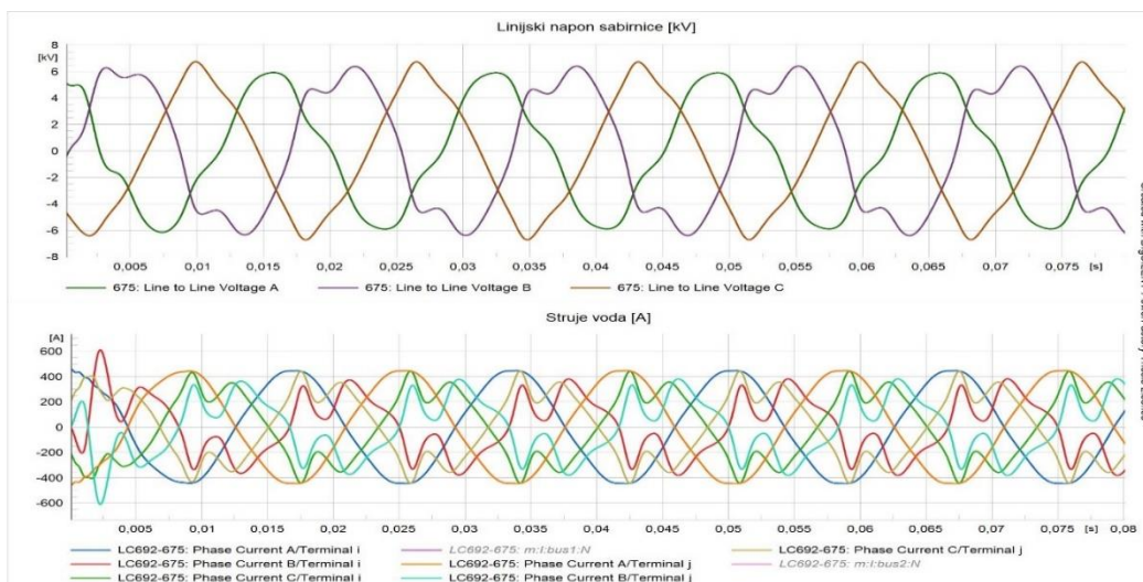
Slika 6.100 Prikaz valnog oblika linijskog napona na sabirnici 675 i struja na ulazu i izlazu voda LC692-675 poslije integracije punionica
