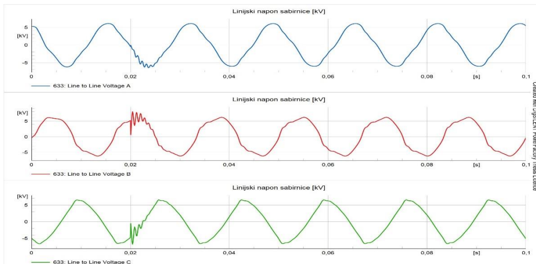
Slika 6.114 Prikaz linijskog napona sabirnice 633 nakon uključanja punionica
