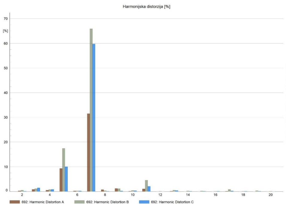
Slika 6.25 Prikaz udjela viših harmonika po fazama sabirnice 692
