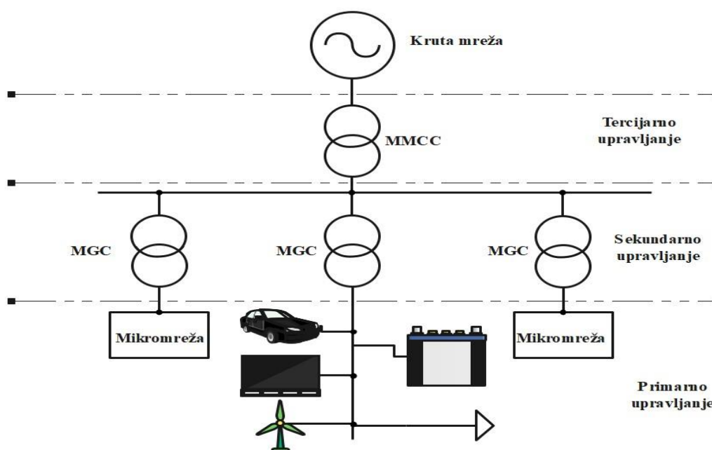
Slika 3.7 Struktura upravljanja mnogostrukih mikromreža [20]
