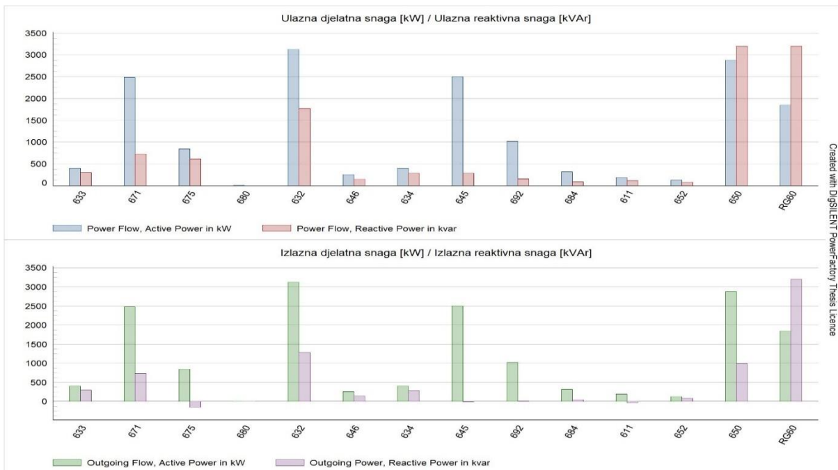
Slika 6.15 Prikaz ulaznih i izlaznih snaga na sabirnicama sustava prije integracije OIE
