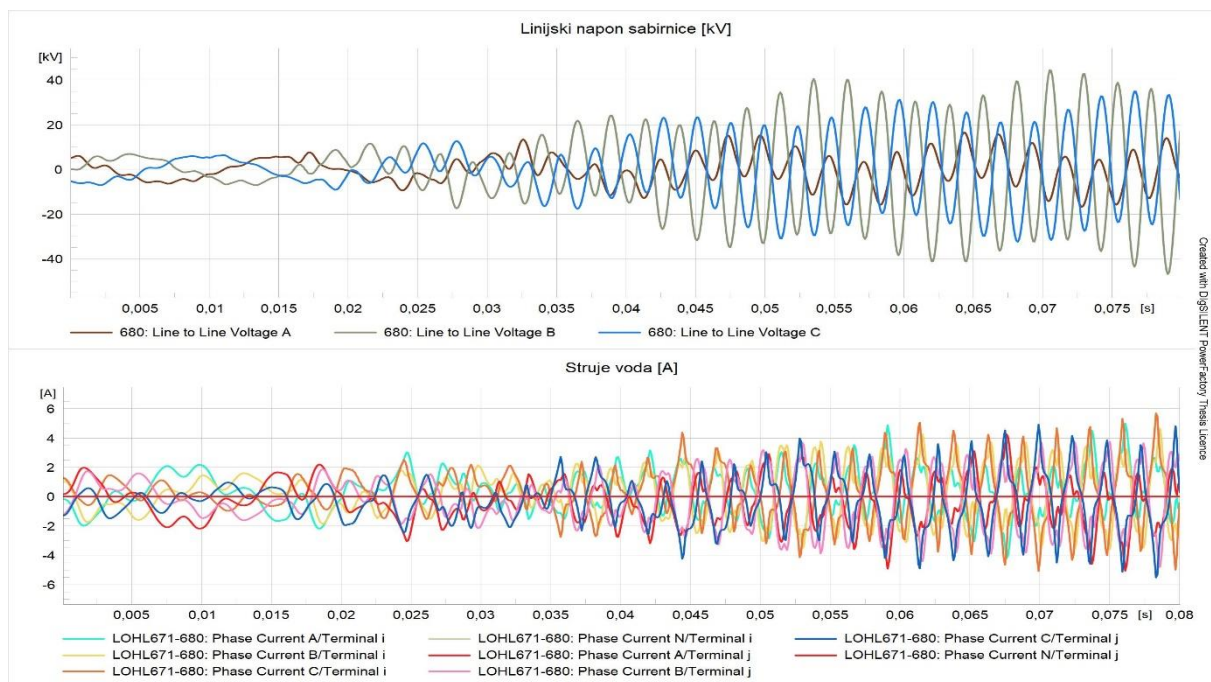
Slika 6.41 Prikaz valnog oblika linijskog napona na sabirnici 680 i struja na ulazu i izlazu voda LOHL671-680 poslije integracije OIE
