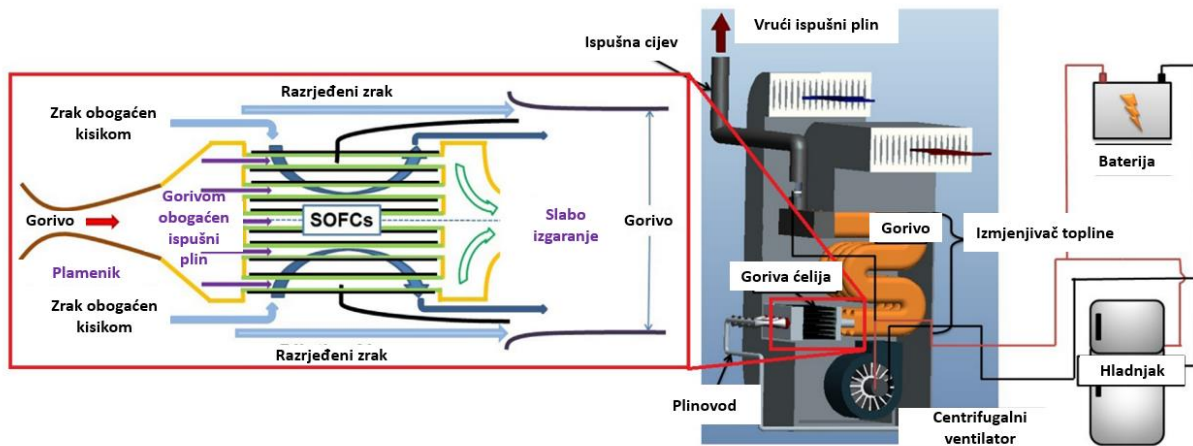
Slika 4.2.3. mCHP jedinica pogonjena sa gorivom ćelijom [34].
