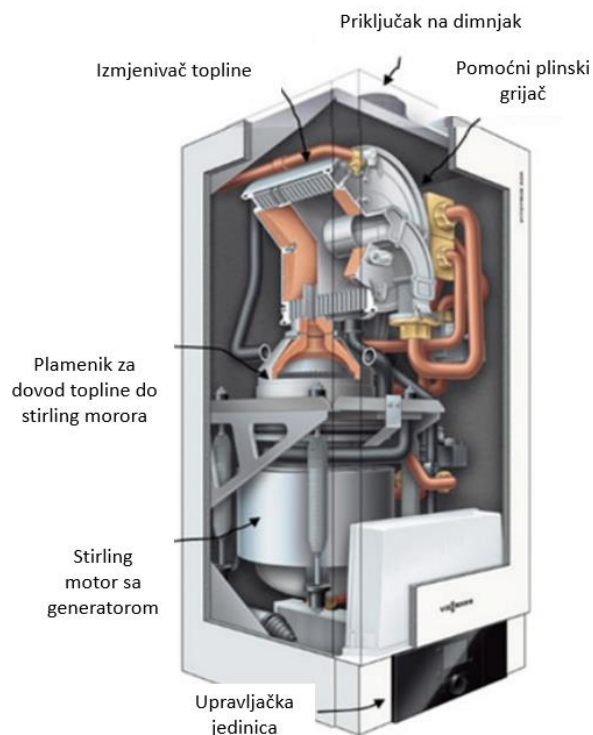
Slika 4.2.4. mCHP jedinica sa Stirling motorom [15].
