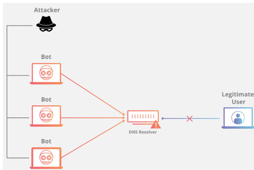
Slika 5.21: DNS flood [16]
