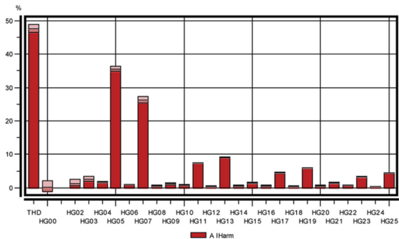
Slika 2.7. Struja i harmonijski spektar 6-pulsnog ispravljača [15]
