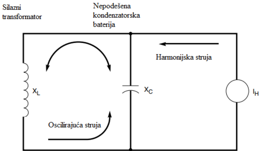
Slika 2.10. Prikaz paralelnog rezonantnog kruga [1]
