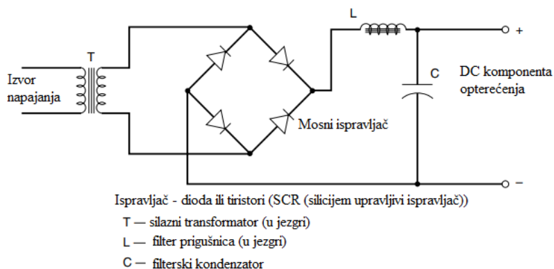
Slika 2.5. Napajanje bez uključenog sklopnog napajanja [1]
