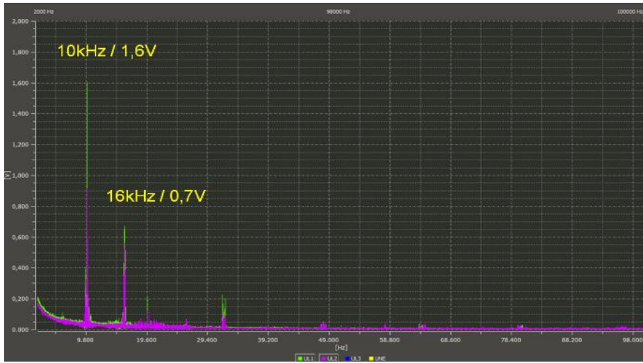
Slika 3.8. prikazuje frekvenciju čopera fotonaponskog invertera i jednog vozila
