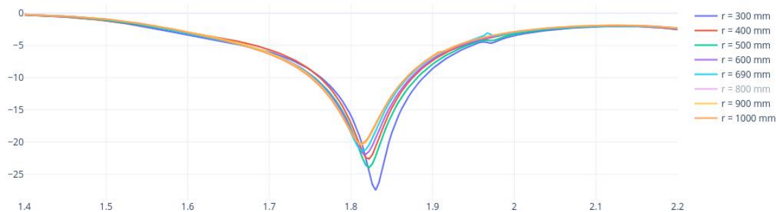
S11 parametar za različite vrijednosti promjera (r) sferne ljsuke antene
