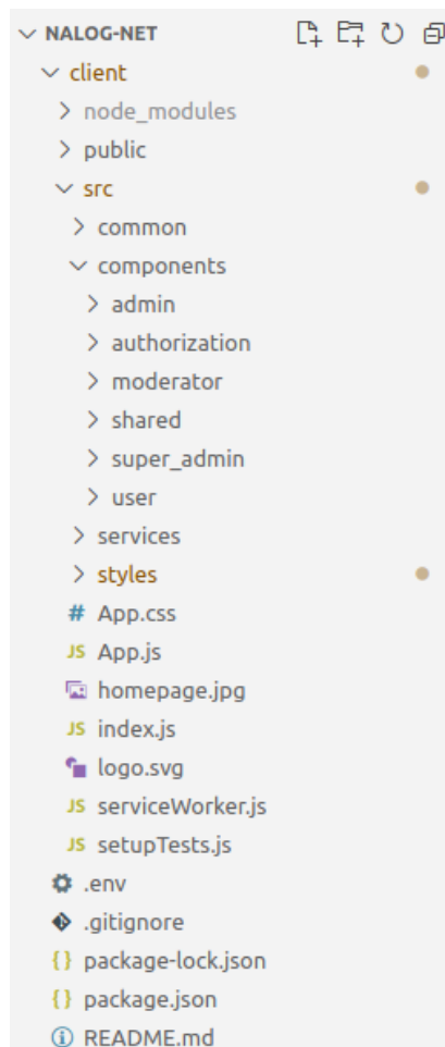
Slika 4.1. Struktura klijenta
