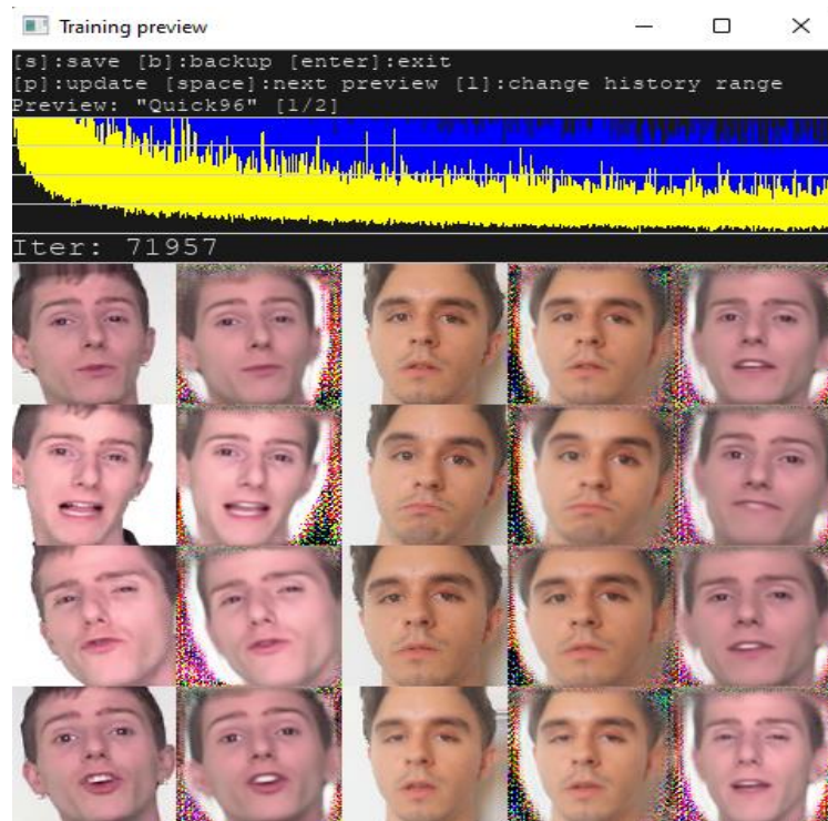
Slika 5.6. Kraj iteriranja
