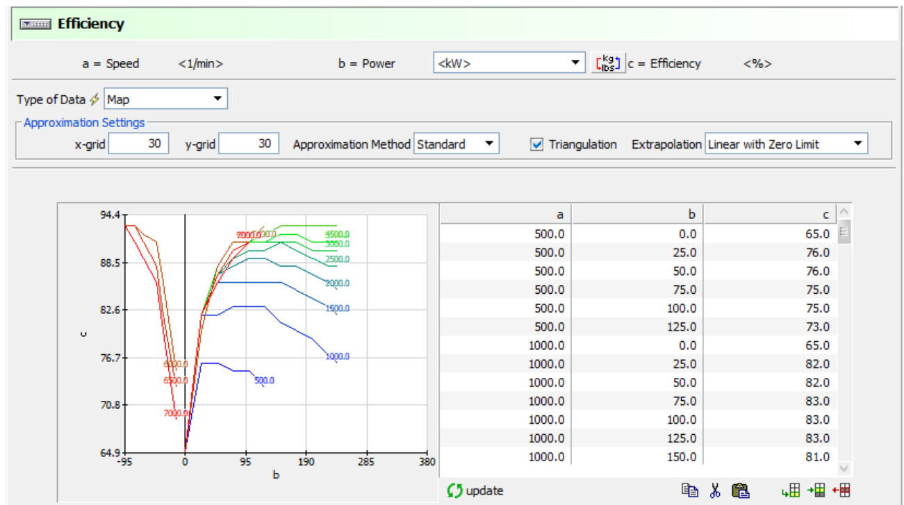
Slika 5.2. Dijagram učinkovitosti elektromotora
