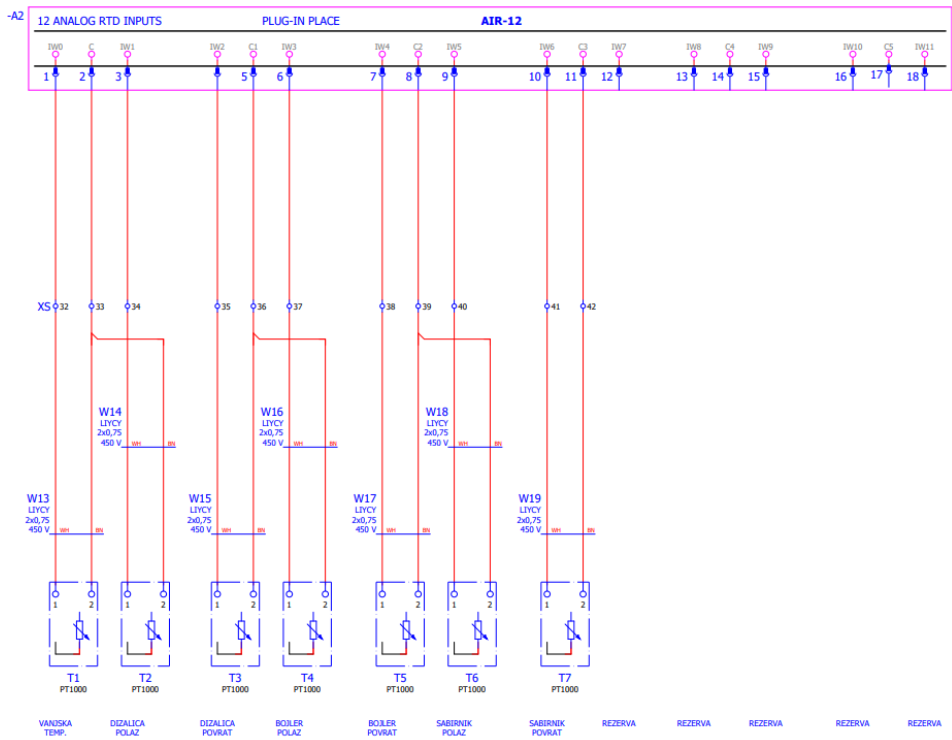
Slika 4.20 Shema spajanja PT1000 sondi - 12 analogni RTD inputi [6]
