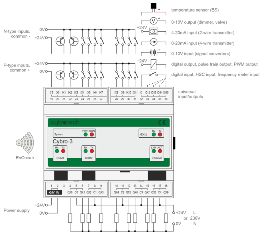
Slika 4.21 Cybrotech CYBRO 3-24 [6]
