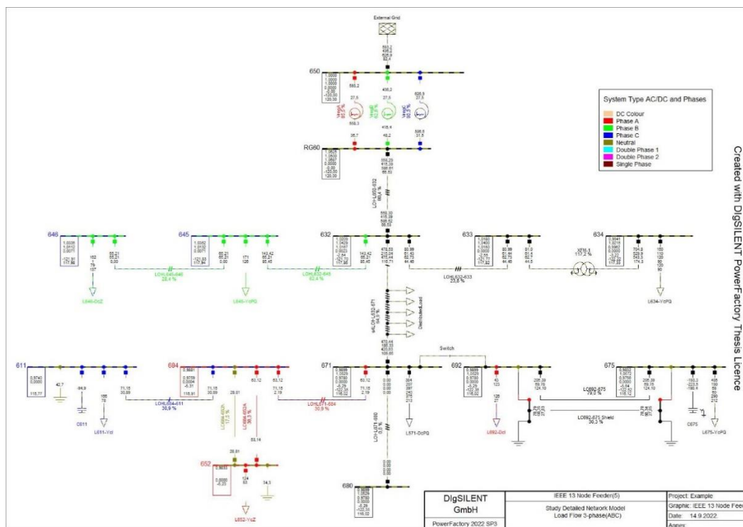
Slika 5.2 Prikaz tokova snaga za prije uključjenja malog industrijskog postrojenja
