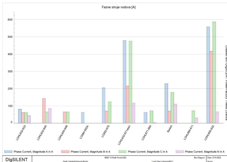
Slika 5.5 Prikaz fazne struja u vodovima mreže
