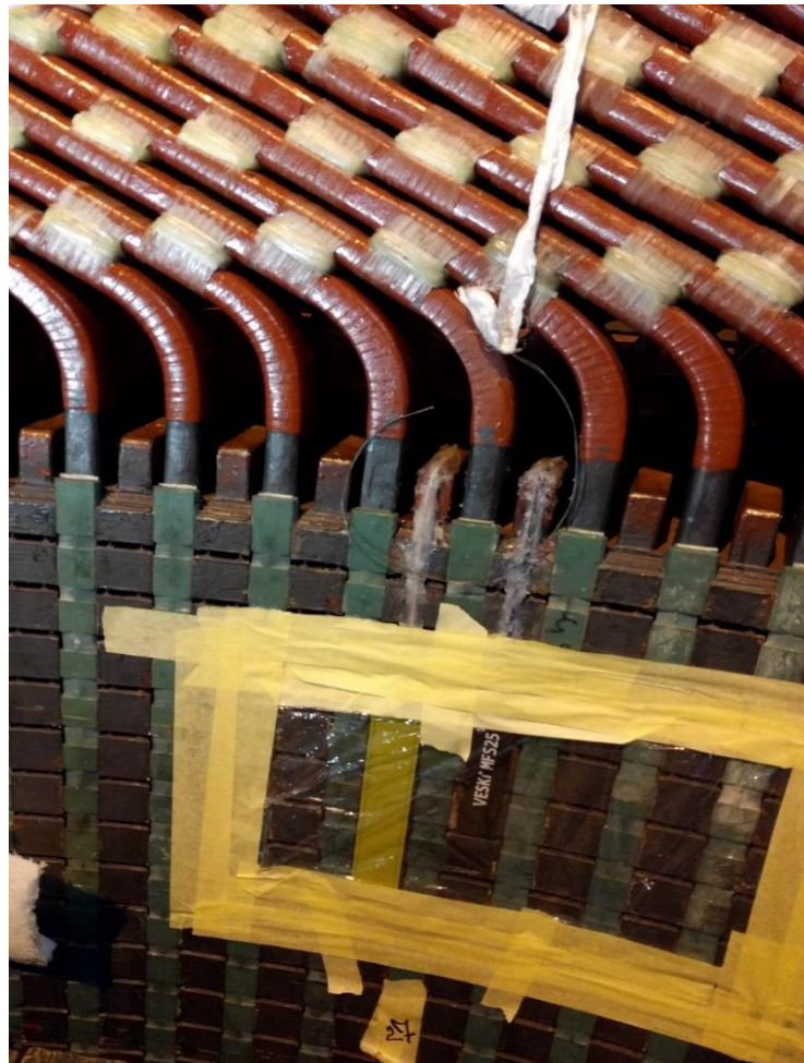
Slika 4.1. Pozicioniranje senzora magnetske indukcije
