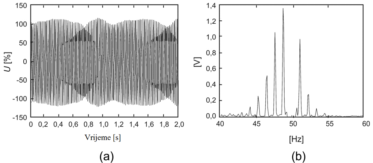
Slika 2.6. a) kolebanje napona na priključcima elektromotora velike snage s promjenjivim opterećenjem b) spektar amplitude moduliranog napona [4]
