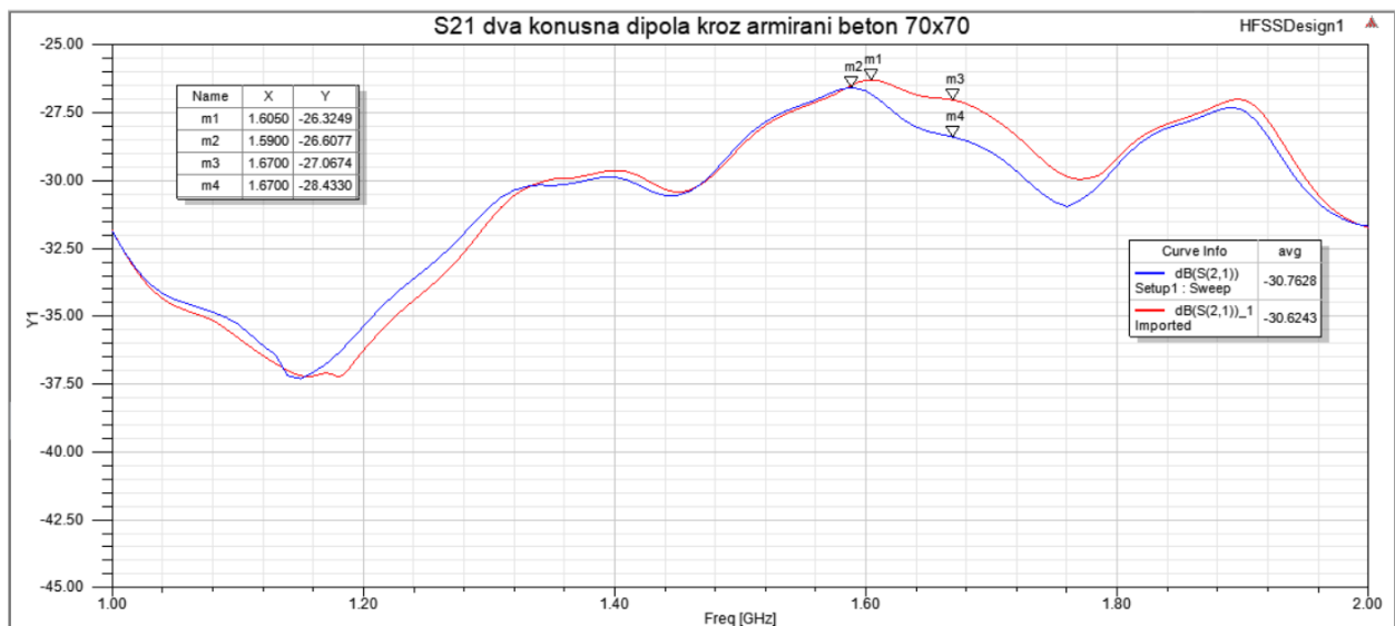
Slika 5.70. Koeficijent transmisije S_{21} kroz prepreku od armiranog betona sa dimenzijom rešetke 70 \times 70 , debljine 8 mm (plava krivulja) i 10 mm (crvena krivulja) u frekvencijskom opsegu 1-2 GHz
