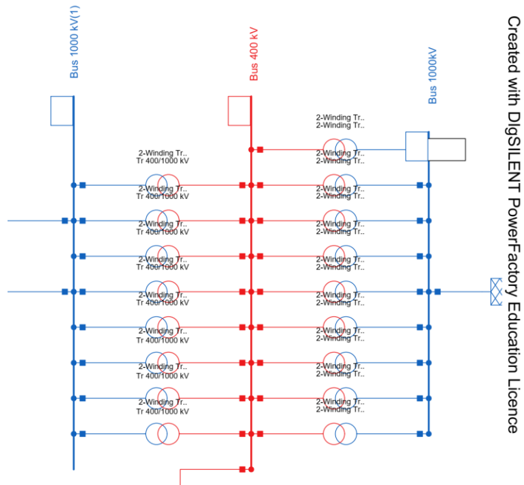
Slika 6.3a. Jednopolna shema VFT sustava sa strane krute mreže
