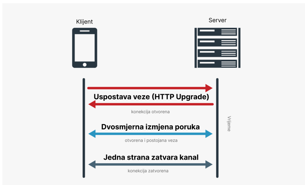
Sl. 3.8. Vizualizacija WebSocket komunikacije
