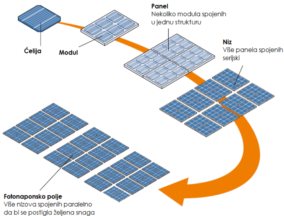
Sl.2.6. Terminologija naziva od ćelije do fotonaponskog polja [5]
