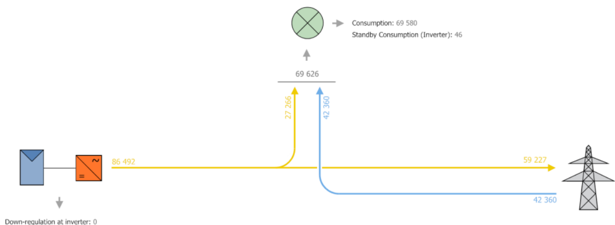
Slika 5.17. Tokovi energije
