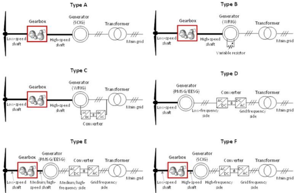
Slika 3.6 Sheme spoja tipova konfiguracije pogonskih sklopova vjetroturbina [14]
