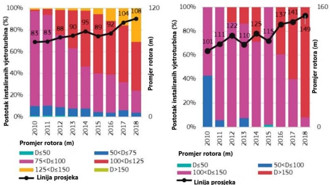
Slika 3.4 Usporedba promjera rotora vjetroturbina na kopnu (lijevo) i pučini (desno) [14]
