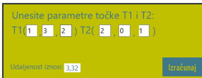
Slika 5.13. Izračun problema udaljenost između dvije točke
