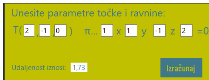
Slika 5.12. Izračun problema udaljenost točke od ravnine
