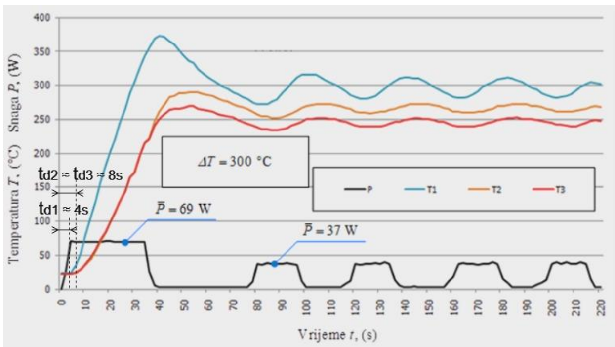
Slika 7.2. Mrtva vremena lemne stanice Weller WE-1010 pri zagrijavanju lemne stanice na temperaturu od 300 \text{ }^\circ\text{C}
