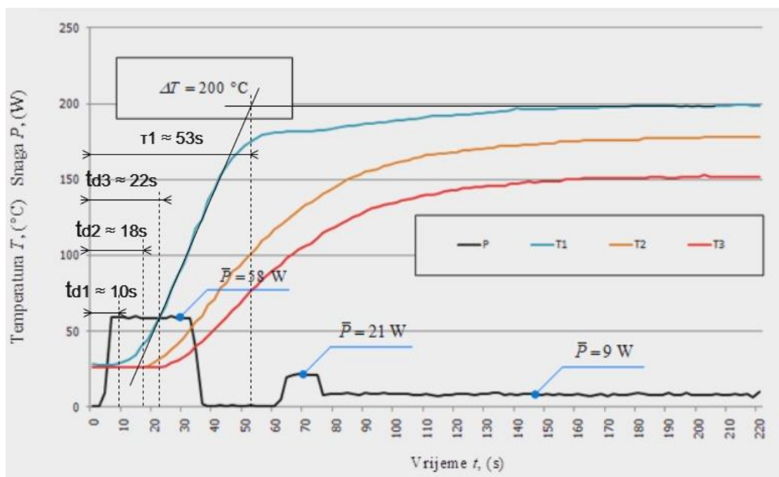
Slika 7.3. Mrtva vremena i vrijeme postizanja ustaljenog stanja lemne stanice Conrad Electronic LSL-450 pri zagrijavanju na temperaturu od 200 \text{ }^\circ\text{C}
