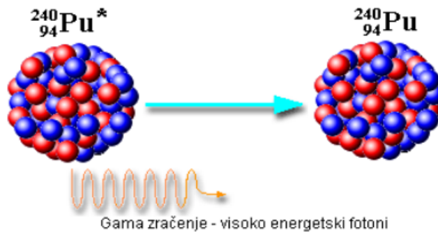
Slika 2.7. Gama zračenje Pu-240
