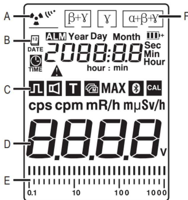
Slika 5.3. Zaslon Geigerovog mjerača zračenja
