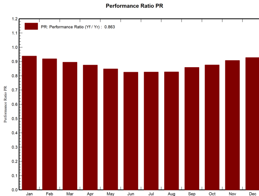
Slika 4.9. Stupanj korisnosti sustava
