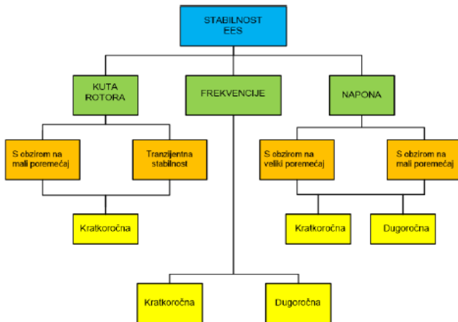
Slika 3.9. Pokazatelji stabilnosti elektroenergetskog sustava [7]
