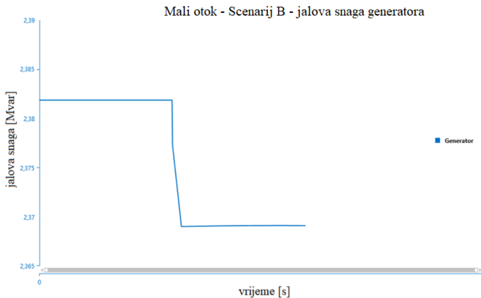
Slika 4.12. Prikaz promjene jalove snage generatora (Mali otok – Scenarij B)
