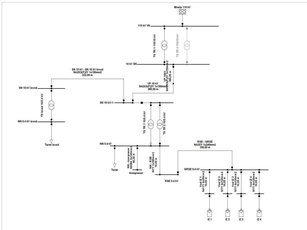
Slika 4.1. Model mreže
