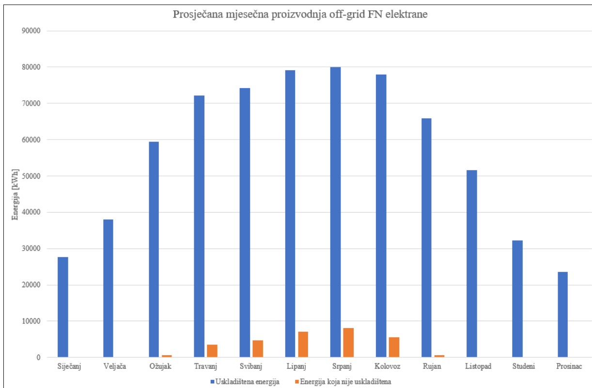
Slika 6.10. Prosječna mjesečna proizvodnja 20 kW off-grid FN elektrane
