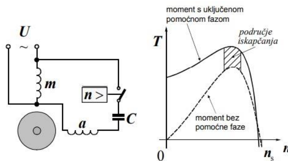
Slika 2.3. Shema spoja i karakteristika momenta asinkronog motora[2]
