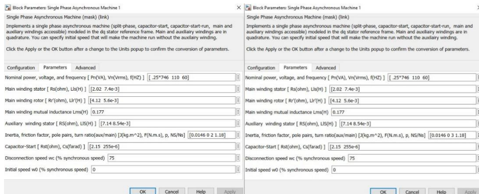
Slika 2.5. Promjena parametra broja pari polova na motorima
