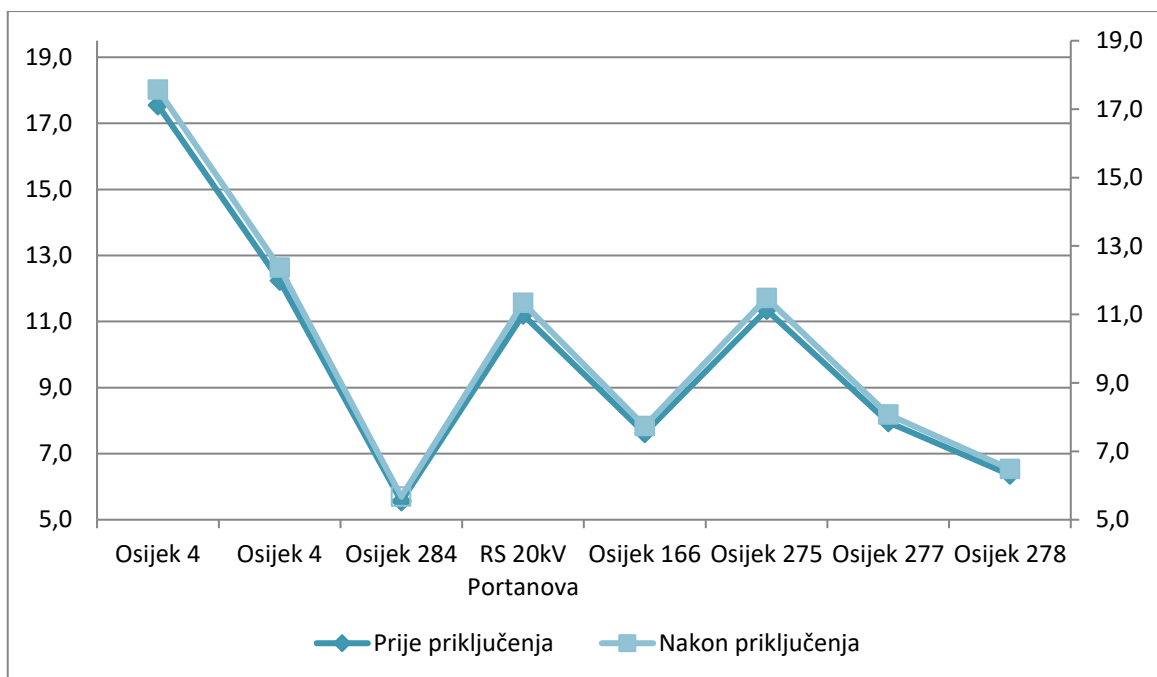
Slika 5.10. Grafički prikaz iznosa struja trolejnog kratkog spoja
