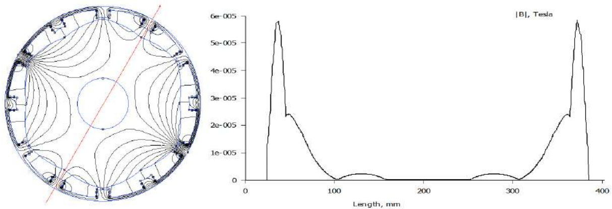
Slika 4.10. Prikaz raspodjele magnetske indukcije duž promjera senzora (pri struji uzbuđnog namota od 0.0083 mA)
